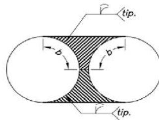
DETALLE SOLDADURA BILATERAL
