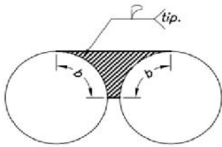
DETALLE SOLDADURA UNILATERAL
